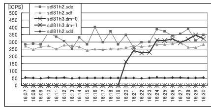
図 9 RAID グループ 1 への I/O 数 (開発方式)
