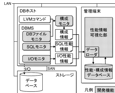
図2 I/O 性能障害診断支援ツールの実装 Fig. 2 Implementation of Diagnostic Tool.
