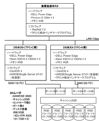
図 3 ハードウェア構成
