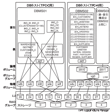
図4 データ配置 Fig. 4 Data mapping.
