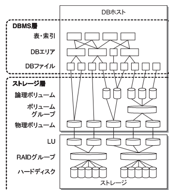
図 1 ストレージおよび DBMS 階層 Fig. 1 Storage and DBMS hierarchy.
