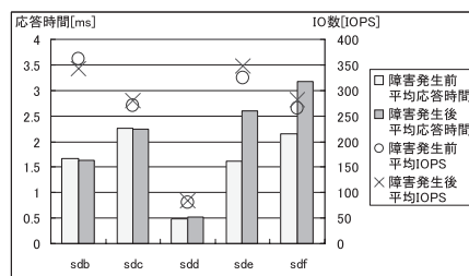
図 7 物理ボリューム別応答時間および IO 数
