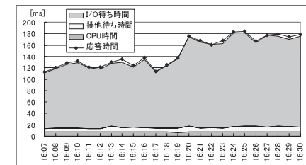
図5 トランザクション応答時間内訳 (従来方式) Fig. 5 Transaction response (conventional).
