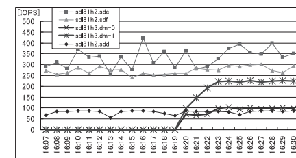
図 8 RAID グループ 1 への I/O 数 (従来方式)
