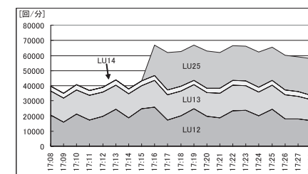
図 13 LU 別 I/O 数 (RAID グループ 1) (従来方式)
