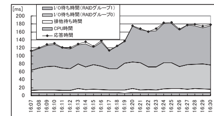
図6 トランザクション応答時間内訳 (開発方式) Fig. 6 Transaction response (developed).
