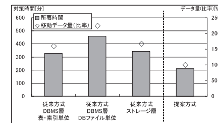
図 15 対策時間およびデータ移動量
