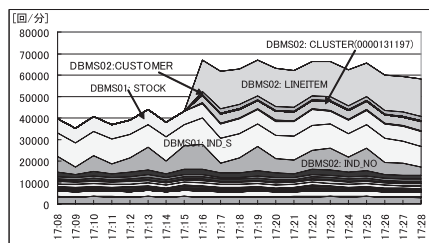
図 14 DBMS の表・索引別 I/O 数 (開発方式)
