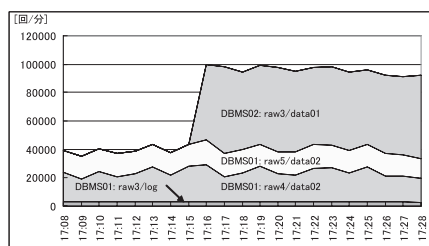
図 12 DB ファイル別 I/O 数 (従来方式)
