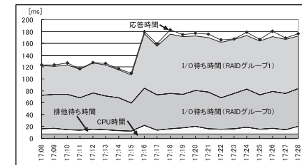
図 10 トランザクション応答時間内訳 (開発方式)
