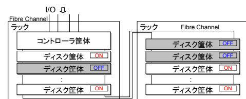
図2 DIASのストレージ装置の概要
