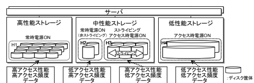
図4 ストレージ階層とデータの配置
