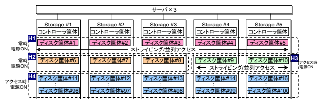
図 6 DIAS のストレージ階層
