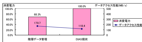
図 11 新規データ追加後の消費電力とアクセス性能
