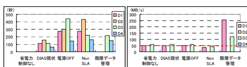
図 8 アクセス待ち時間(左)及びアクセス性能(右)
