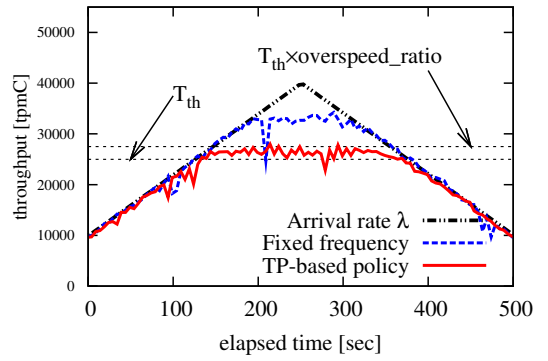
図 6 到着率とスループットの時間変化
