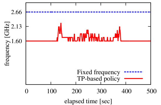
図 7 動作周波数の時間関係
