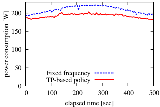
図 8 消費電力の時間関係
