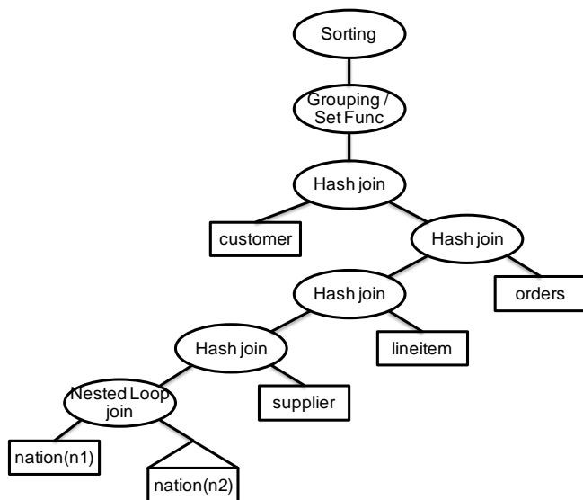
図 8 Q7 実行プラン
