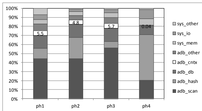
図 10 Q7 実行時の CPU 処理内訳
