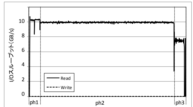
図 5 Q8 実行時の I/O スループット
