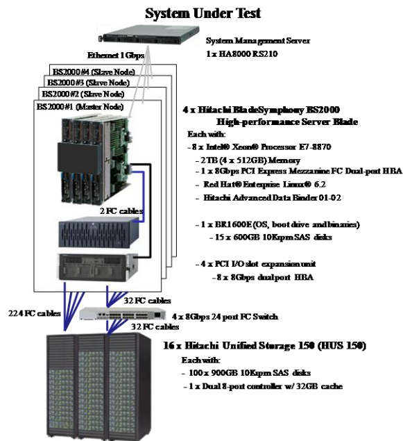
図 2 TPC-H ベンチマーク評価環境
