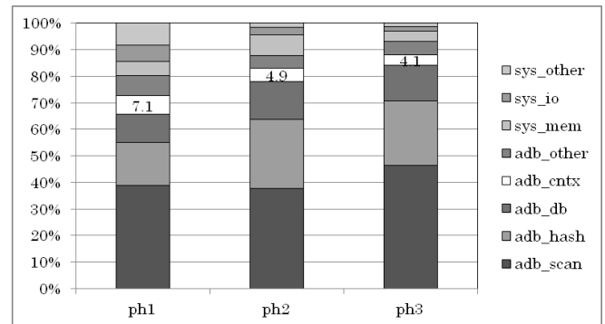
図 6 Q8 実行時の CPU 処理内訳
