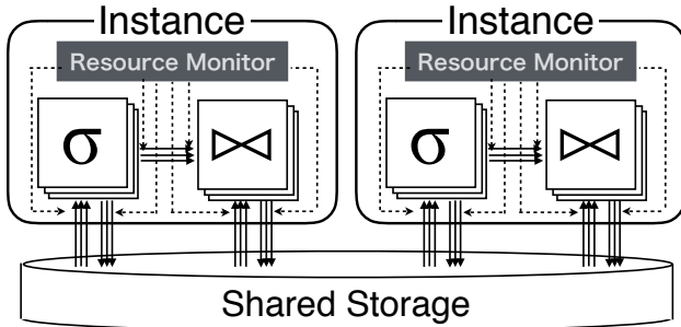
図 4: 共有ストレージ型データベースにおけるリソースモニタ
