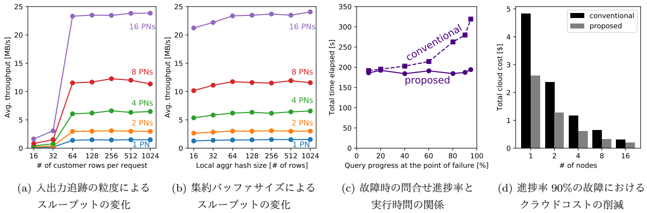
図 4 耐障害型問合せ実行方式の性能特性と動的障害回復の効果
