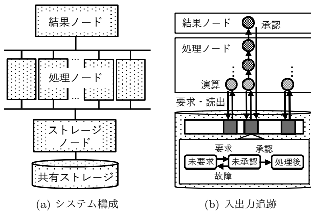
図 1 並列データベースシステムの構成と入出力追跡
