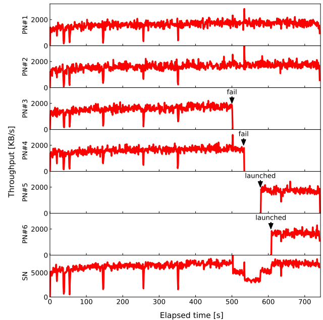
図 3 ノード故障時の動的障害回復の動作挙動。上 6 段が各処理ノード、最下段がストレージノードの挙動を表す。
