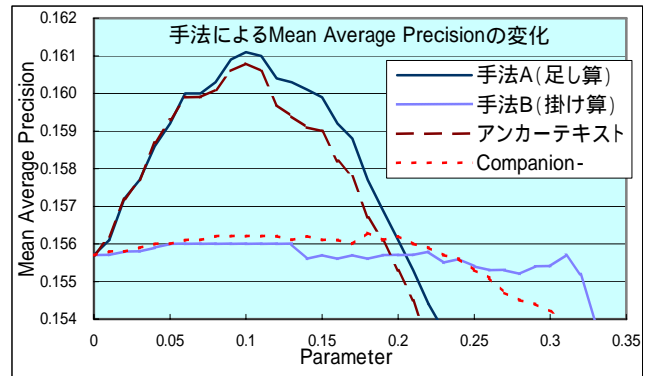
図 3 . アンカーテキストとリンク構造解析の統合手法
