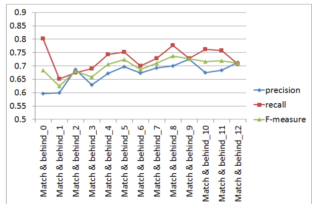
図 9 素性とする形態素数による分類性能 (学習データにおける交差検定)
